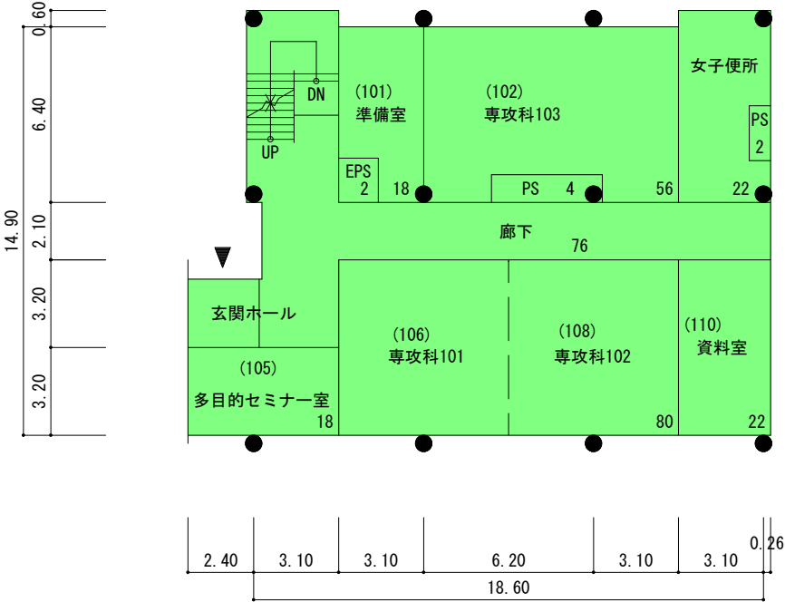
1階平面図 床面積 300㎡ S=1/250
