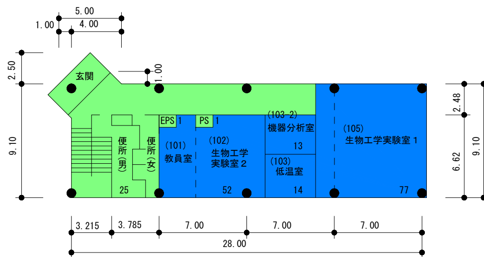
1階平面図 床面積 264㎡
