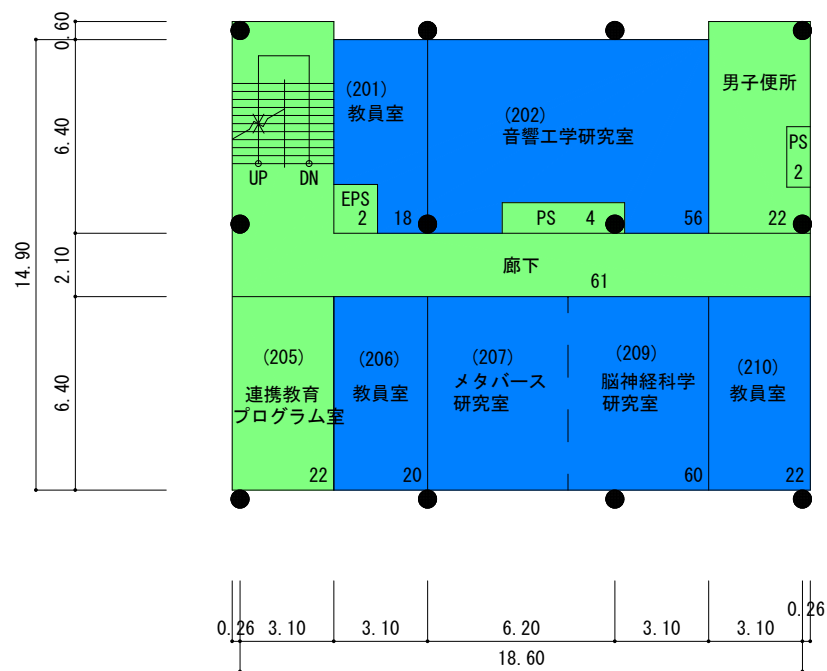
2階平面図 床面積 289㎡ S=1/250
