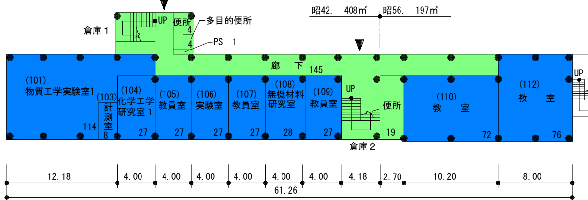
1階 平面図 床面積 605㎡ S=1/400
