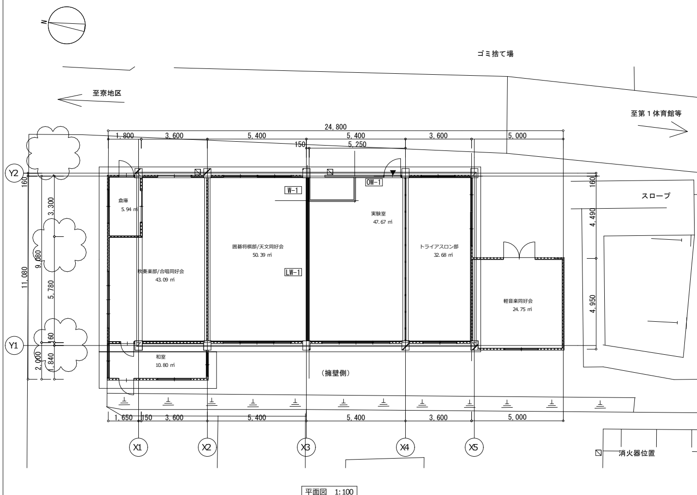
平面图 1:100
