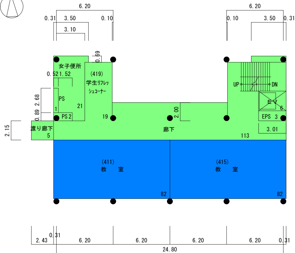
4 階平面図 床面積 334㎡ S=1/250
