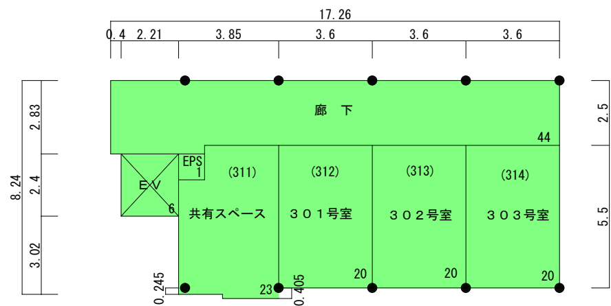
3階平面図 床面積 134m 2 S=1/200
