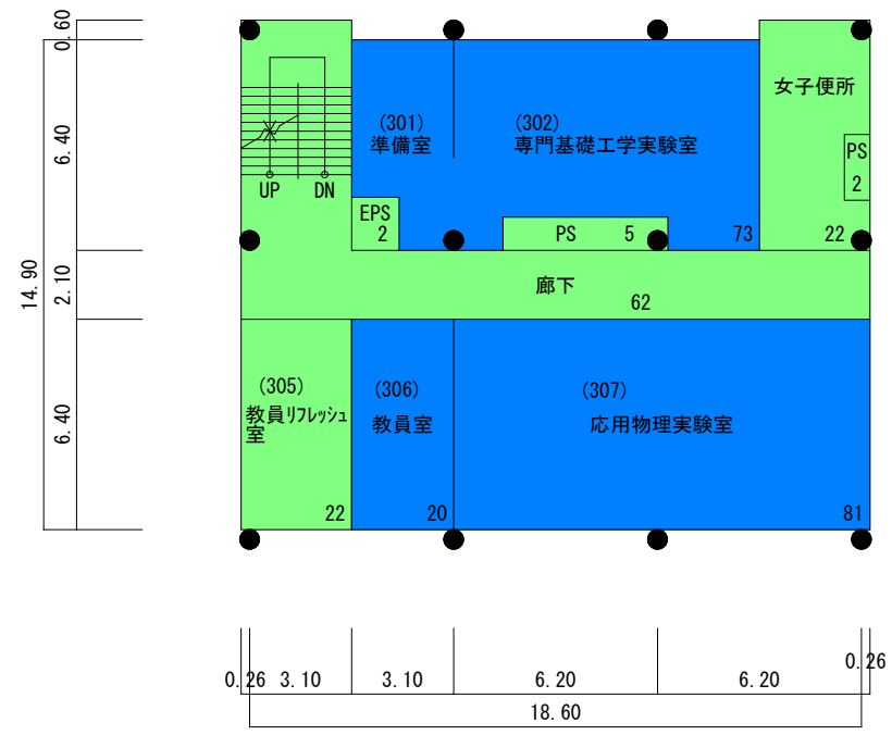
3階平面図 床面積 289㎡ S=1/250
