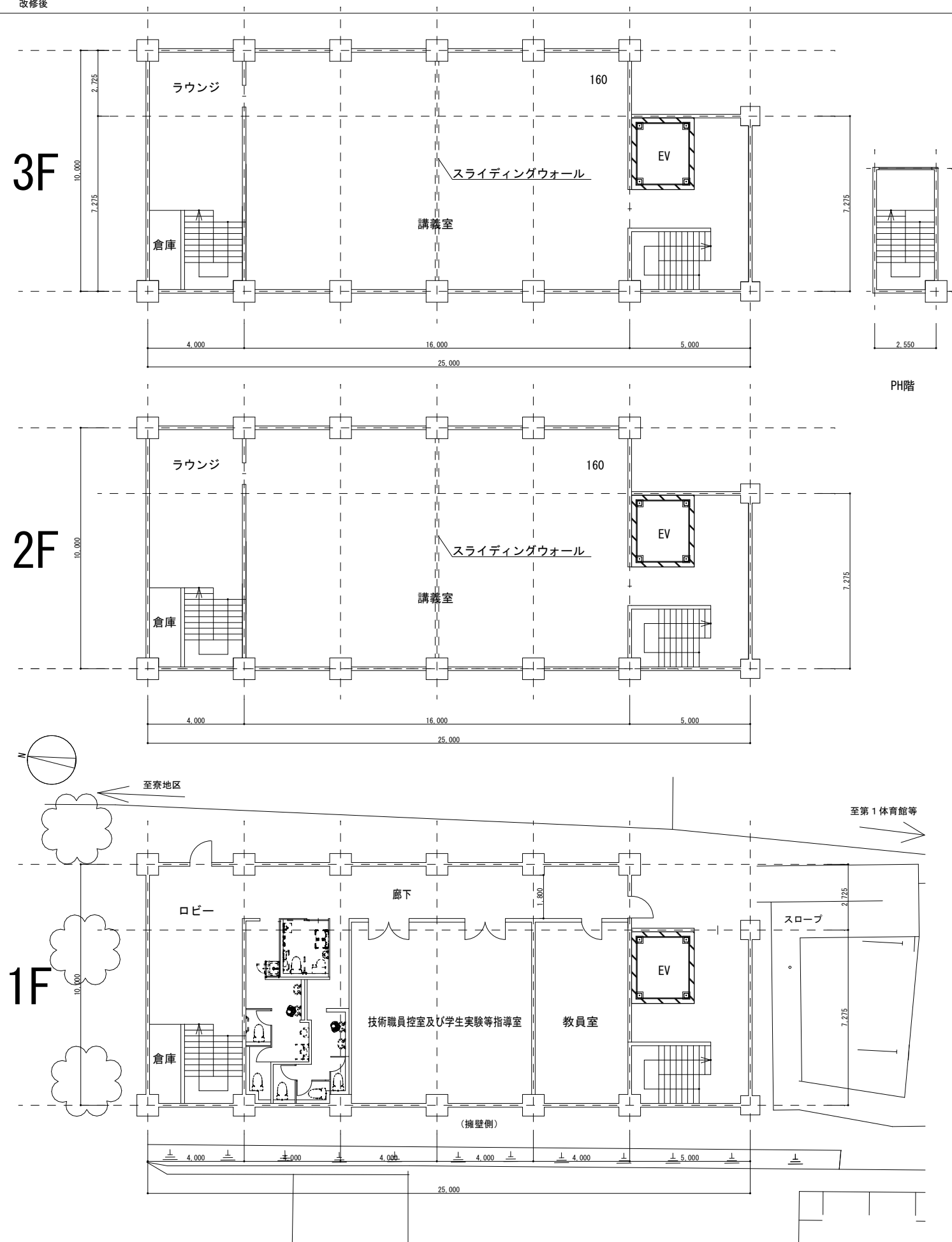
平面图 1:100
