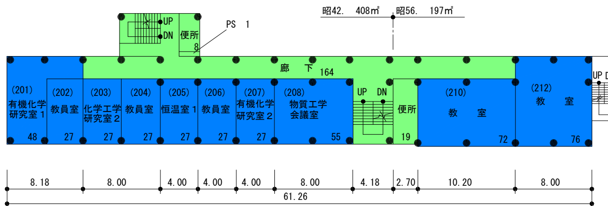
2階 平面図 床面積 605㎡ S=1/400
