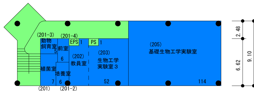
2階平面図 床面積 250㎡
