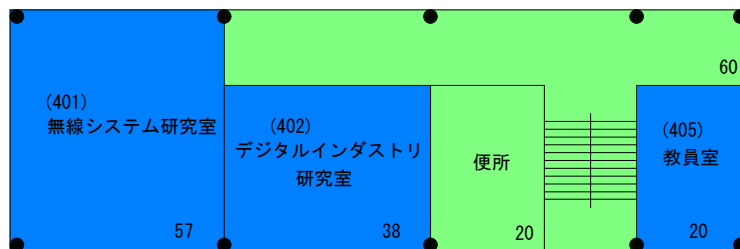
4階平面図 床面積 195㎡ S=1/250
