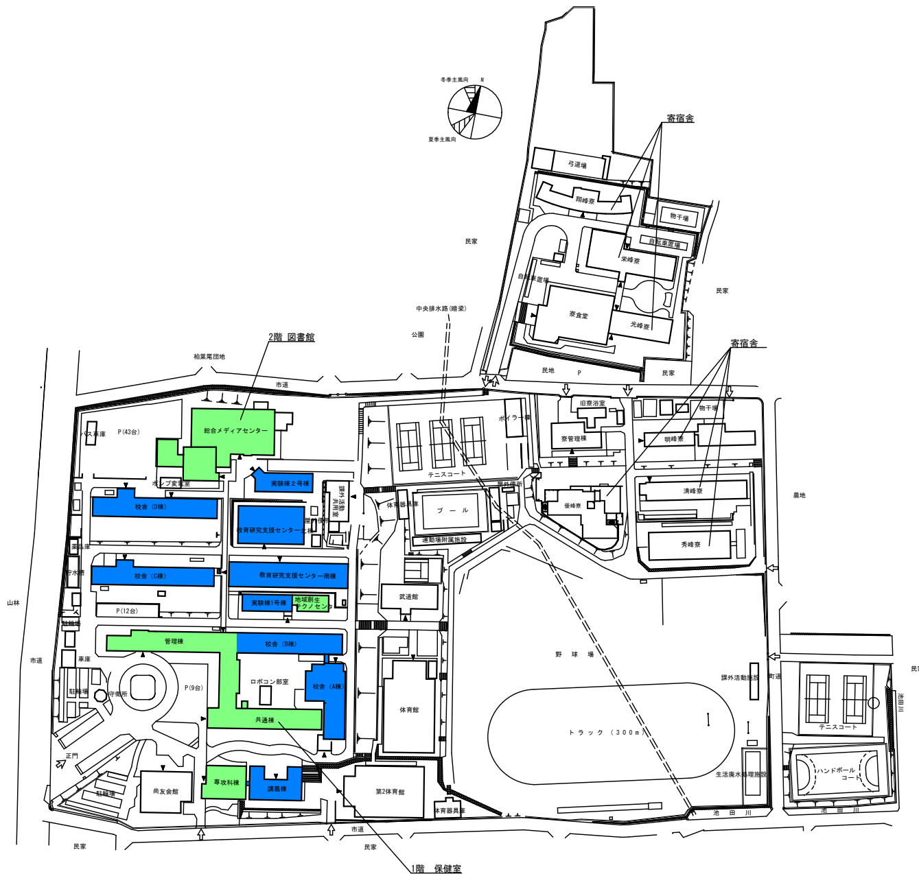
大岡団地配置図 S=1/900 (A1)
