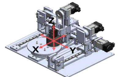
図4 非接触搬送
