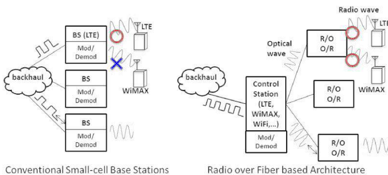
光ファイバ無線を用いた中央一括制御・異種無線システム
