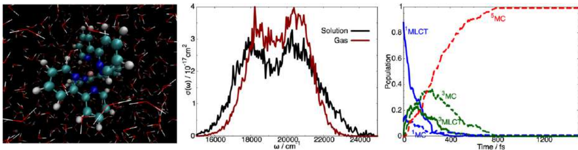
分子動力学シミュレーションにより計算された [\text{Fe}(\text{bpy})_3]^{2+} 水溶液(左図)の吸収スペクトル(中央図)と光励起後の population 変化(右図)。S. Iuchi and N. Koga, J. Phys. Chem. Lett. 14, 4225 (2023).
