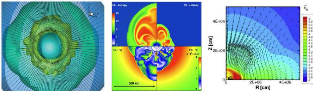
6次元ボルツマン方程式を解く計算コードにより得られた超新星爆発（左、中）および連星中性子星合体（右）における
