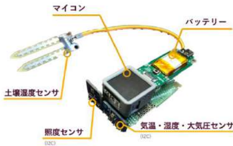
植物生育環境モニタリングのためのエッジデバイス
