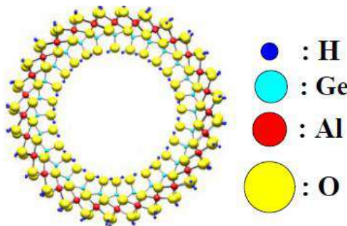
アルミノゲルマネートナノチューブの構造モデル
