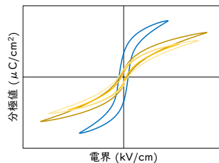
得られた薄膜の電気特性
