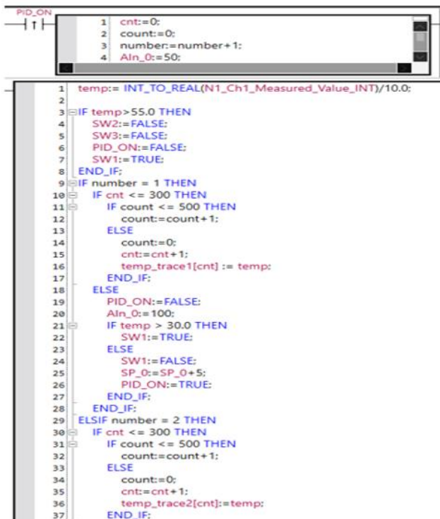
図 6 学生が作成したラダープログラム
