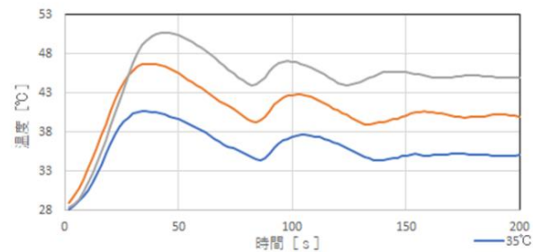
図4 異なる目標値に対するオートチューニング結果
